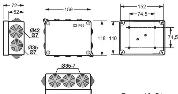
Figura 18. Dimensiones de la caja para montaje
