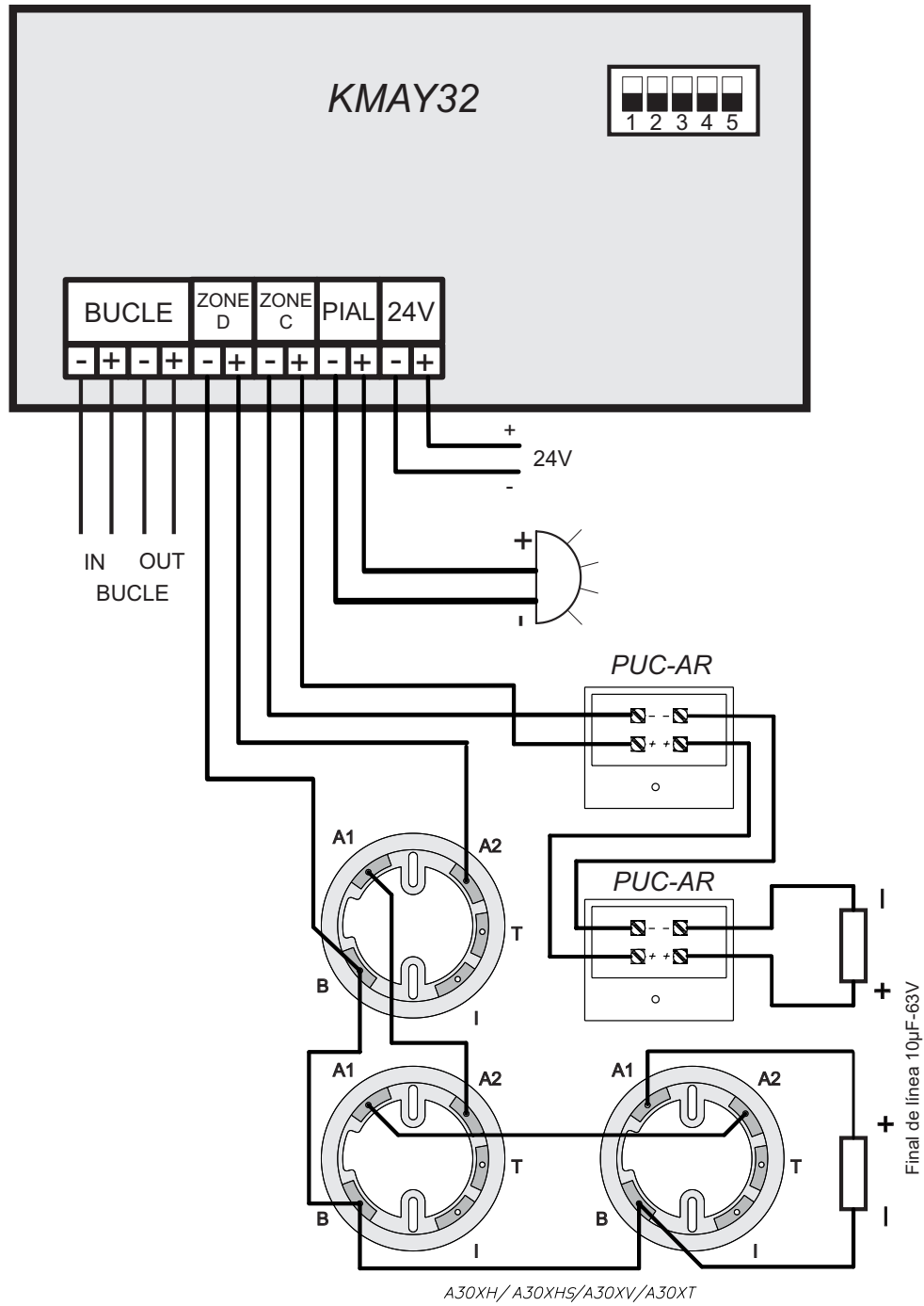
Figura 17. Esquema de conexionado
